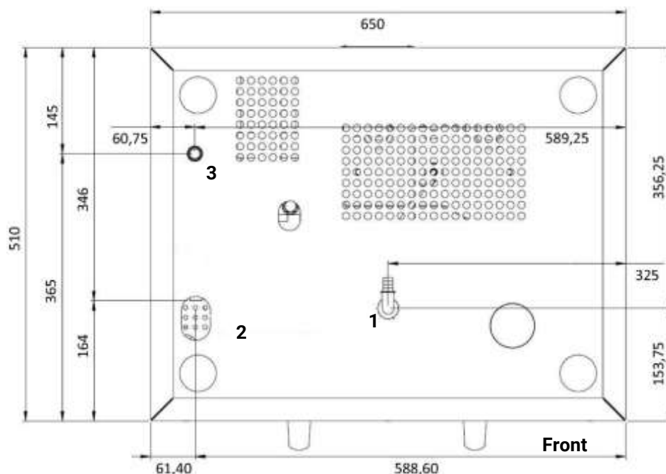
Anschlussplan (Draufsicht)
