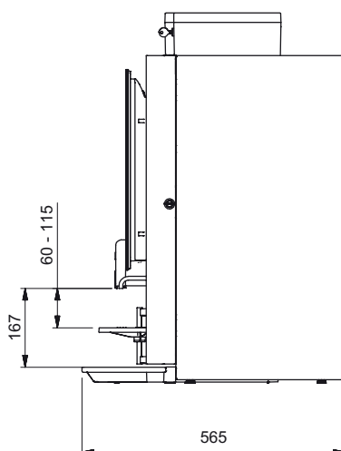
SEITENANSICHT RECHTS
